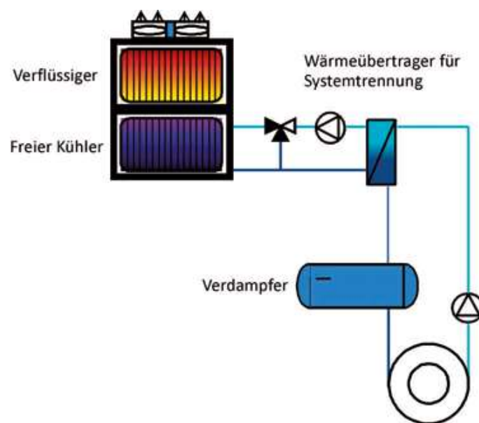
Bild III-9: Hydraulische Funktionsdarstellung: Freie Kühlung mit Systemtrennung durch Wärmeübertrager
